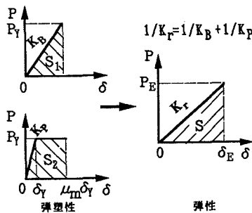
図-2 免震支承を等価線形モデルとした場合の弾塑性応答
